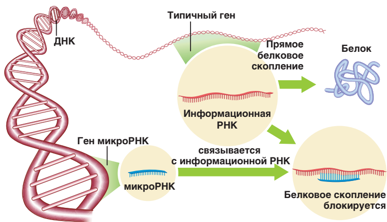
Рис. 1.9. Строение микроРНК
